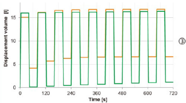
容積變化
