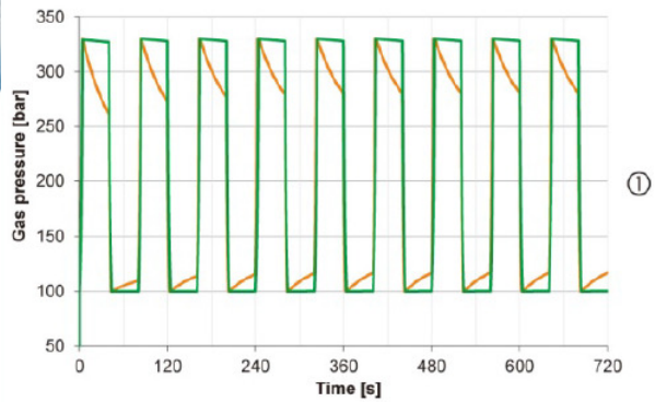
壓力變化
