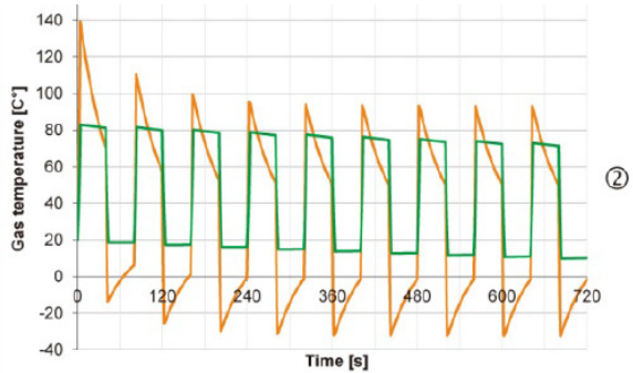
溫度變化
